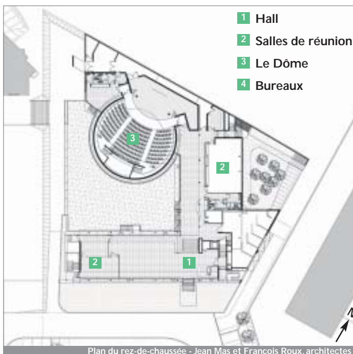
Plan du rez-de-chaussée - Jean Mas et François Roux, architectes
